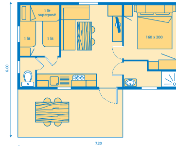
MOBILE HOME AZUR / 5 Plätze - 28 m 2 + Terrasse 10 m 2
